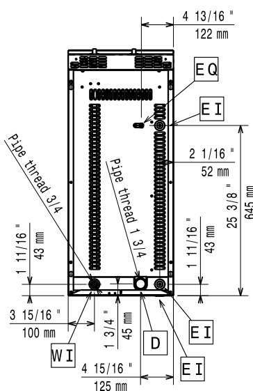
Boven aanzicht
